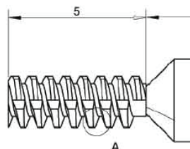
Zahnrad Profilfräser D 2,02 mm
